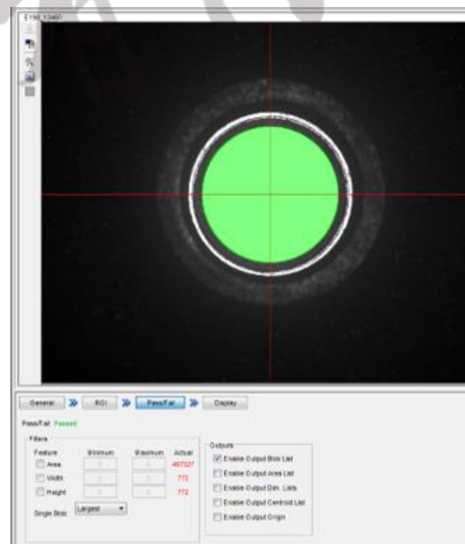
內徑尺寸量測
